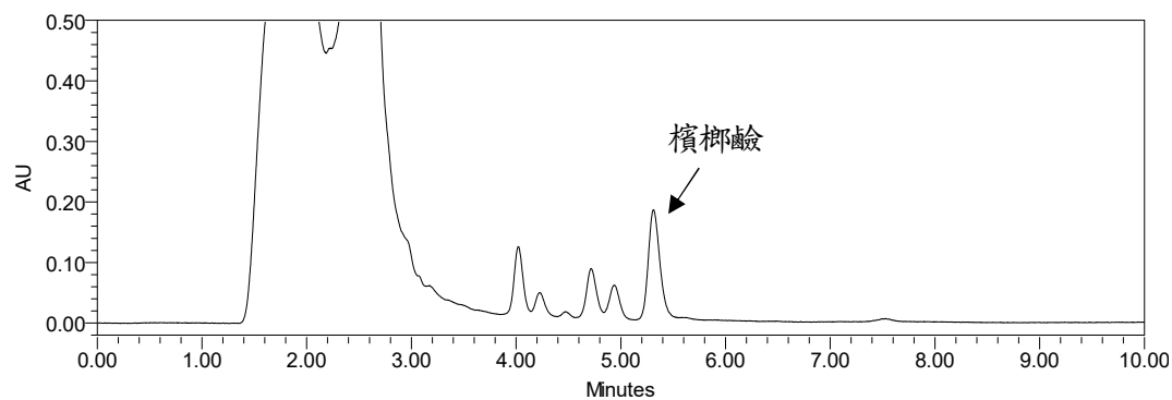
圖八、市售大腹皮藥材檢品之 UPLC 層析圖
