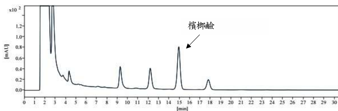
圖二、市售大腹皮藥材檢品之 HPLC 層析圖
