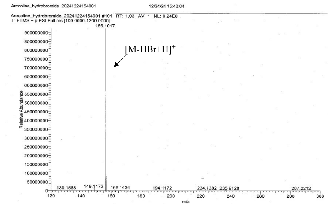
圖十一、氫溴酸檳榔鹼的 ESI-MS 圖譜
