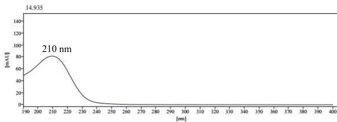
圖十三、氫溴酸檳榔鹼的 UV 圖譜
