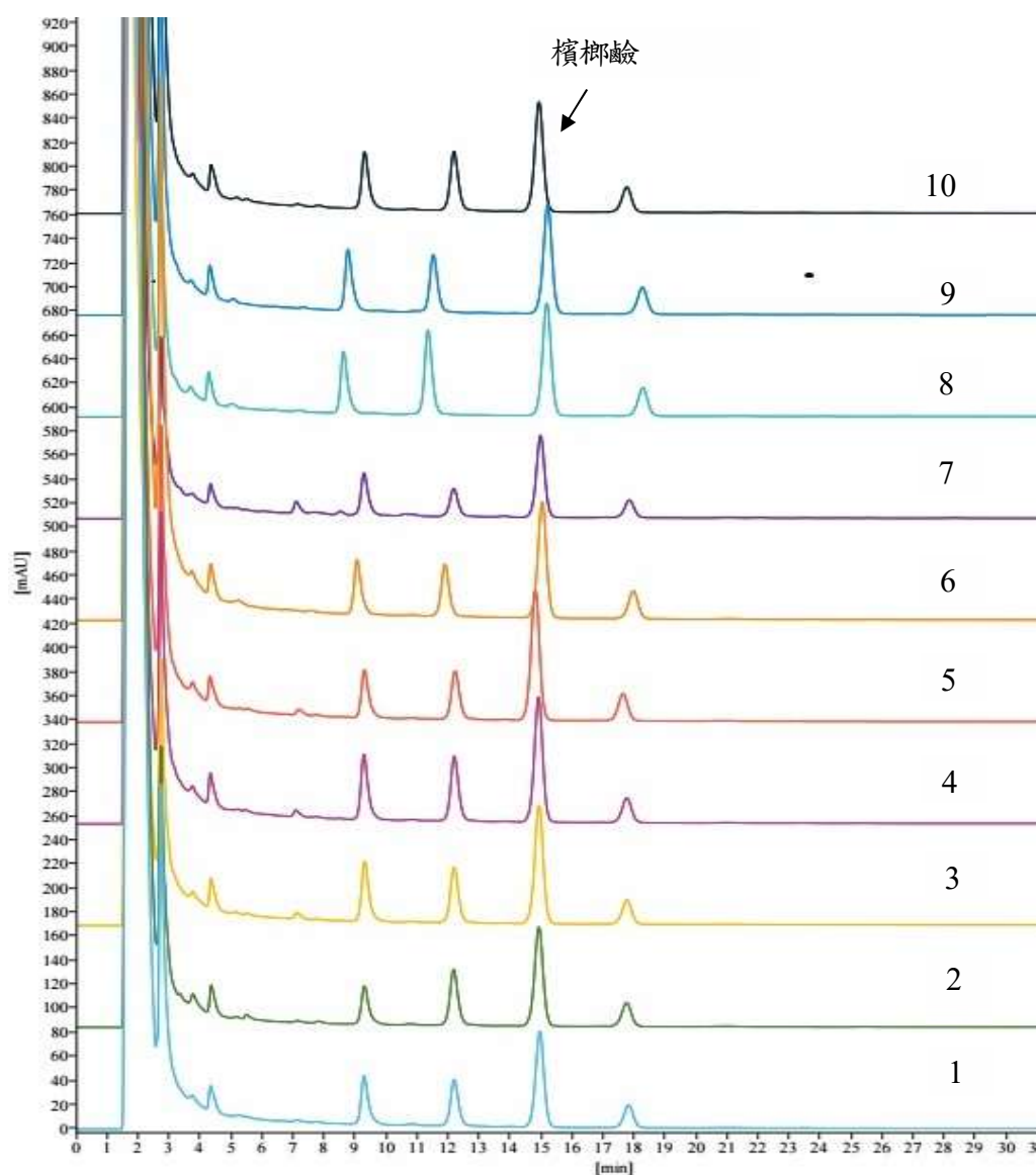
圖六、10 批大腹皮藥材之 HPLC 指紋圖譜
