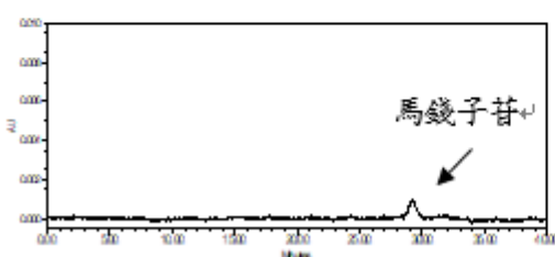
圖八、馬錢子苷之偵測極限層析圖
