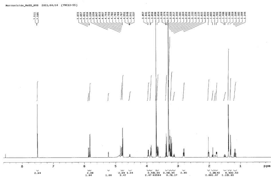
圖十四、莫諾苷的 ^1H NMR 圖譜( CD_3OD )
