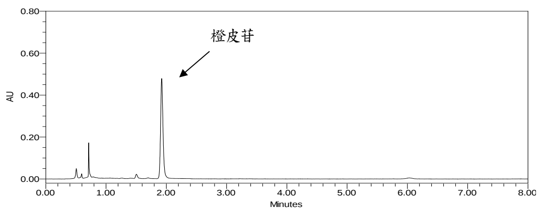
圖七、市售青皮飲片檢品之 UPLC 層析圖
