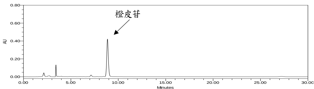
圖二、市售青皮飲片檢品之 HPLC 層析圖
