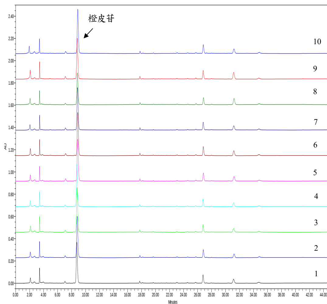
圖六.、10 批青皮藥材之 HPLC 指紋圖譜
