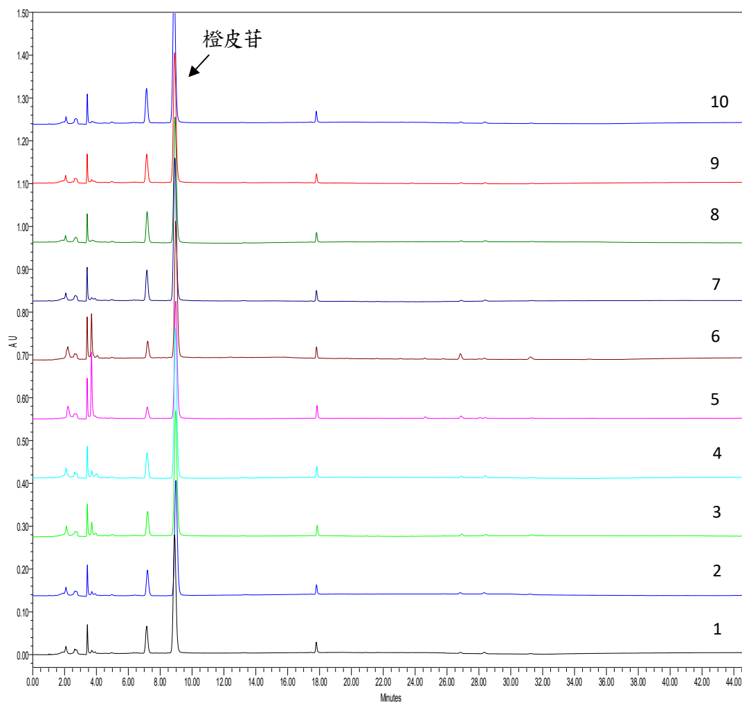
圖六、10 批陳皮藥材之 HPLC 指紋圖譜
