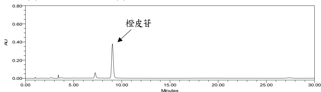
圖二、市售陳皮檢品之 HPLC 層析圖
