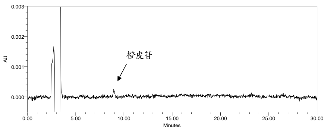
圖四、橙皮苷之偵測極限層析圖
