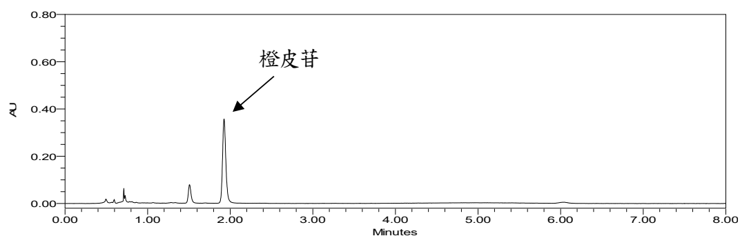
圖八、市售陳皮藥材檢品之 UPLC 層析圖
