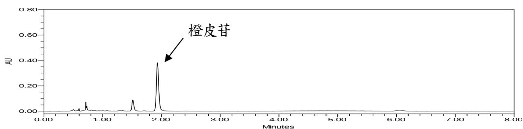
圖七、市售陳皮飲片檢品之 UPLC 層析圖
