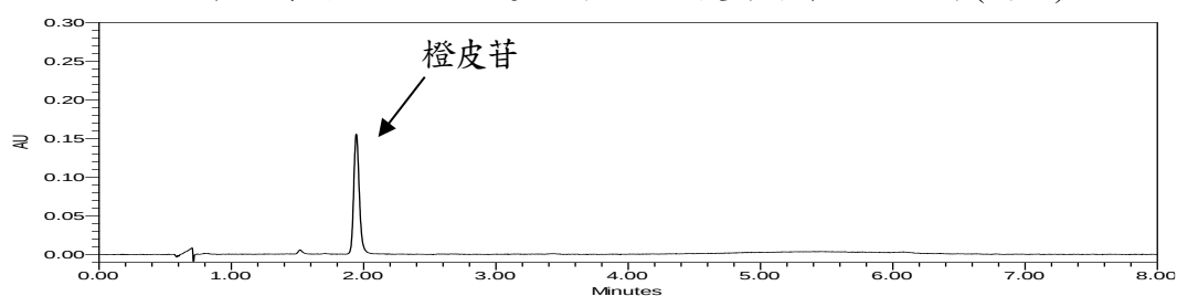
圖六、橙皮苷標準品溶液之 UPLC 層析圖
