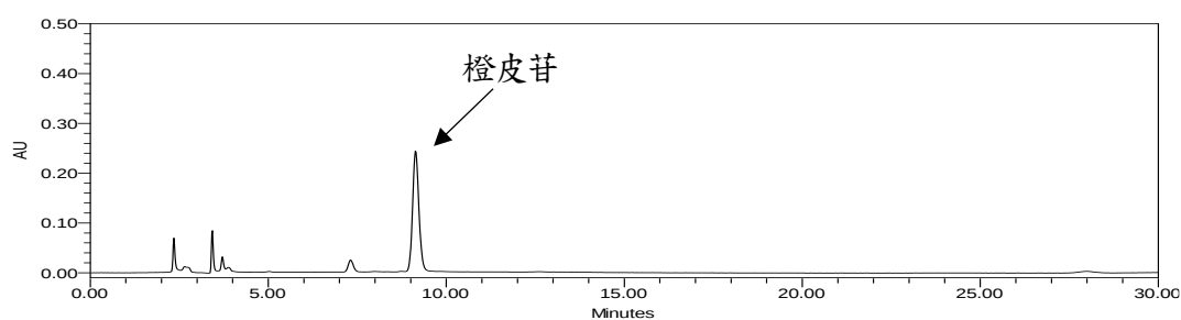
圖二、市售陳皮飲片檢品之 HPLC 層析圖
