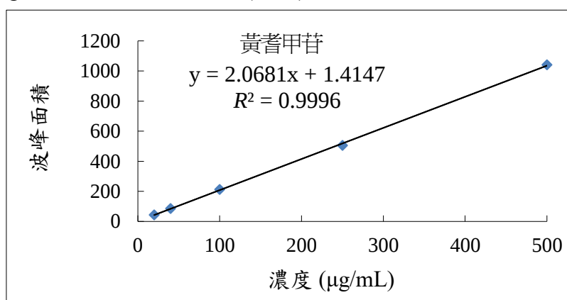
圖三、黃耆甲苷之檢量線圖
