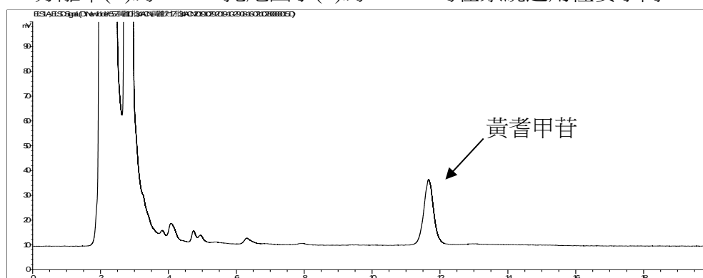
圖二、市售黃耆飲片檢品之 HPLC 層析圖
