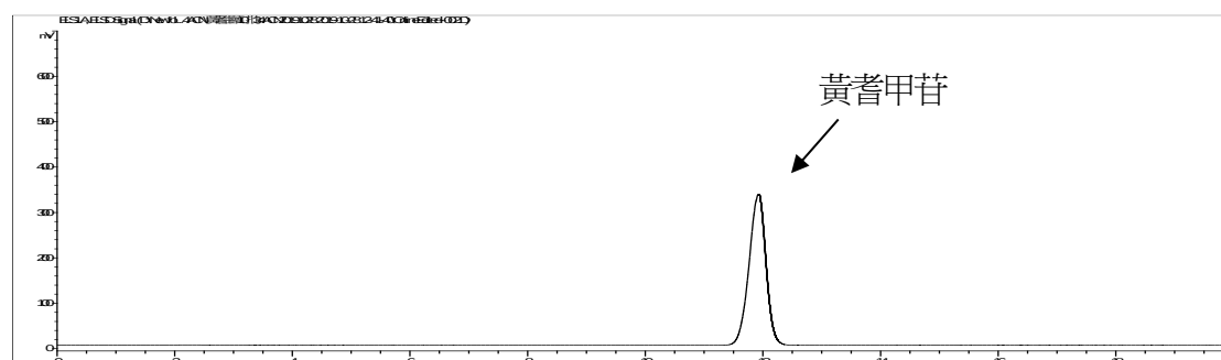
圖一、黃耆甲苷標準品溶液之 HPLC 層析圖
