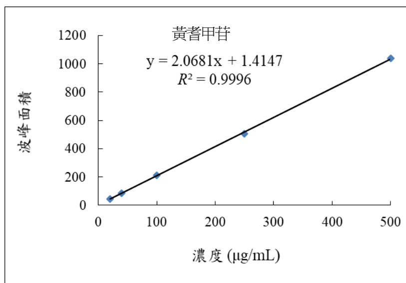
圖三、黃耆甲苷之檢量線圖
