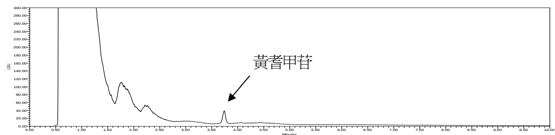
圖八、市售黃耆檢品之 UPLC 層析圖
