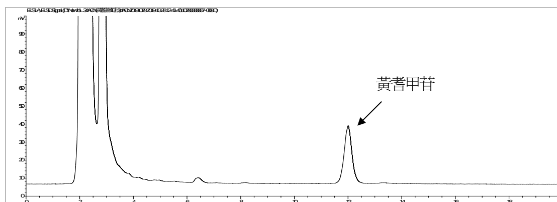
圖二、市售黃耆檢品之 HPLC 層析圖
